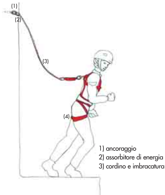
Fig. 11 - Sistema di arresto caduta costituito da imbracatura, cordino e assorbitore di energia
