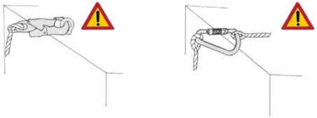
Fig. 15 - Elementi di attacco usati impropriamente
